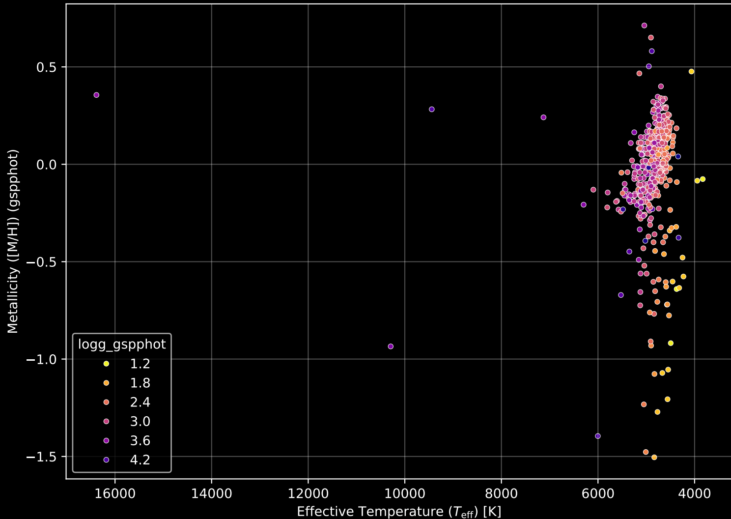
APOGEE DR17 Field: [311-06] Stellar Population Parameters (n= 518)
